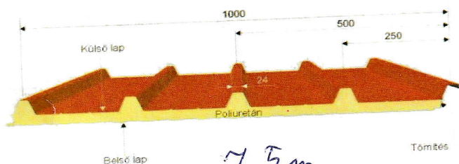
Szendvicspanel tetőre ( PUR töltet )
